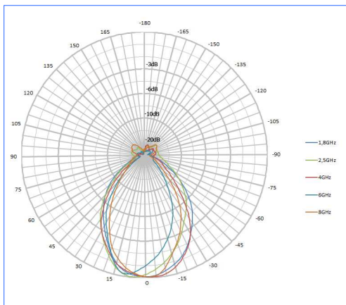
수평 패턴 HyperLOG 30xx Serie
