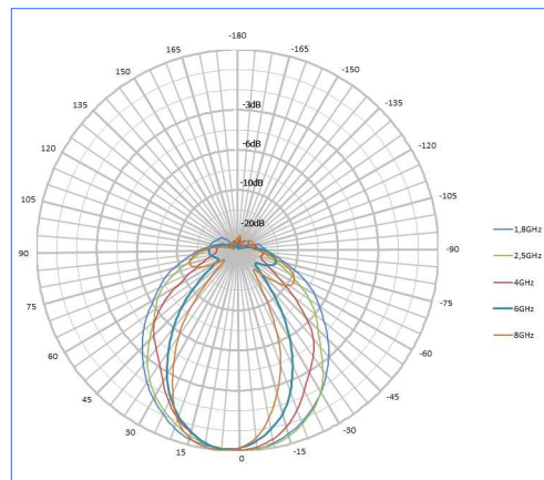
수직 패턴 HyperLOG 30xx Serie
