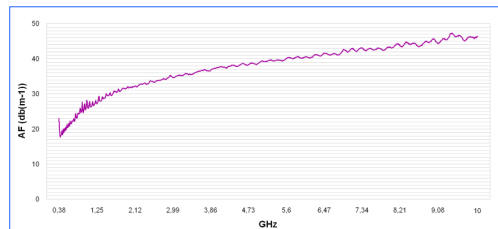
안테나 인수 HyperLOG 30100
