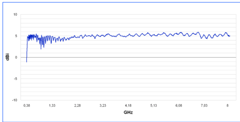
이득 그래프 HyperLOG 3080
