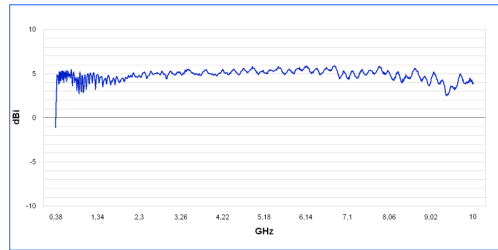
이득 그래프 HyperLOG 30100
