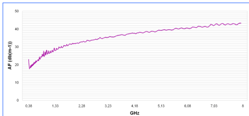
안테나 인수 HyperLOG 3080
